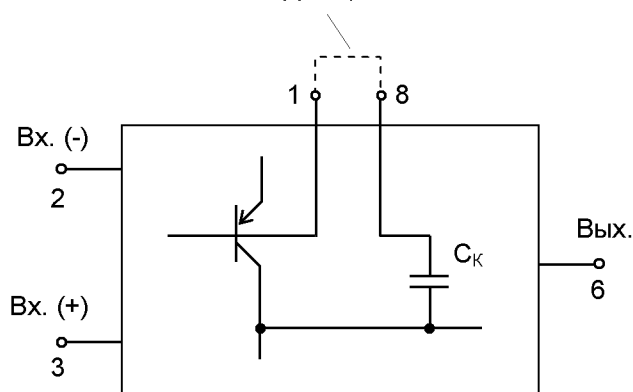
Организация внутренней частотной коррекции 544УД2
