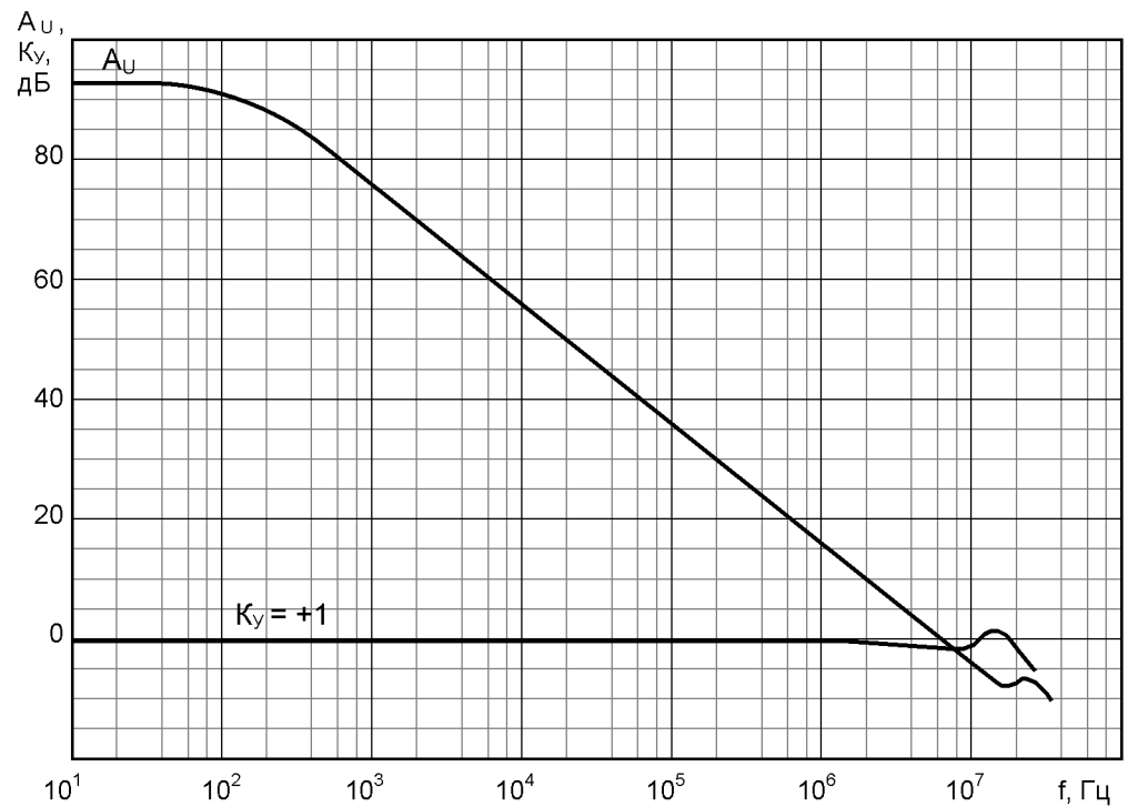
Включение 544УД2 при K_y < 20 и в режиме повторителя напряжения (внутренняя частотная коррекция включена)
