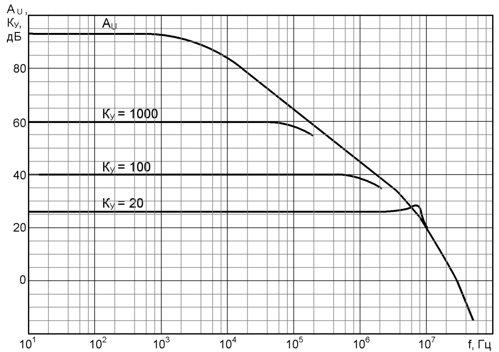
Оптимальное включение 544УД2 при K_y \geq 20 (внутренняя частотная коррекция отключена)
